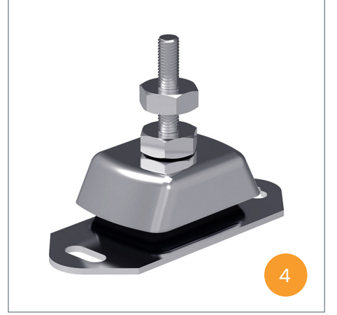
MARİN TİP VİBRASYON TAKOZU
